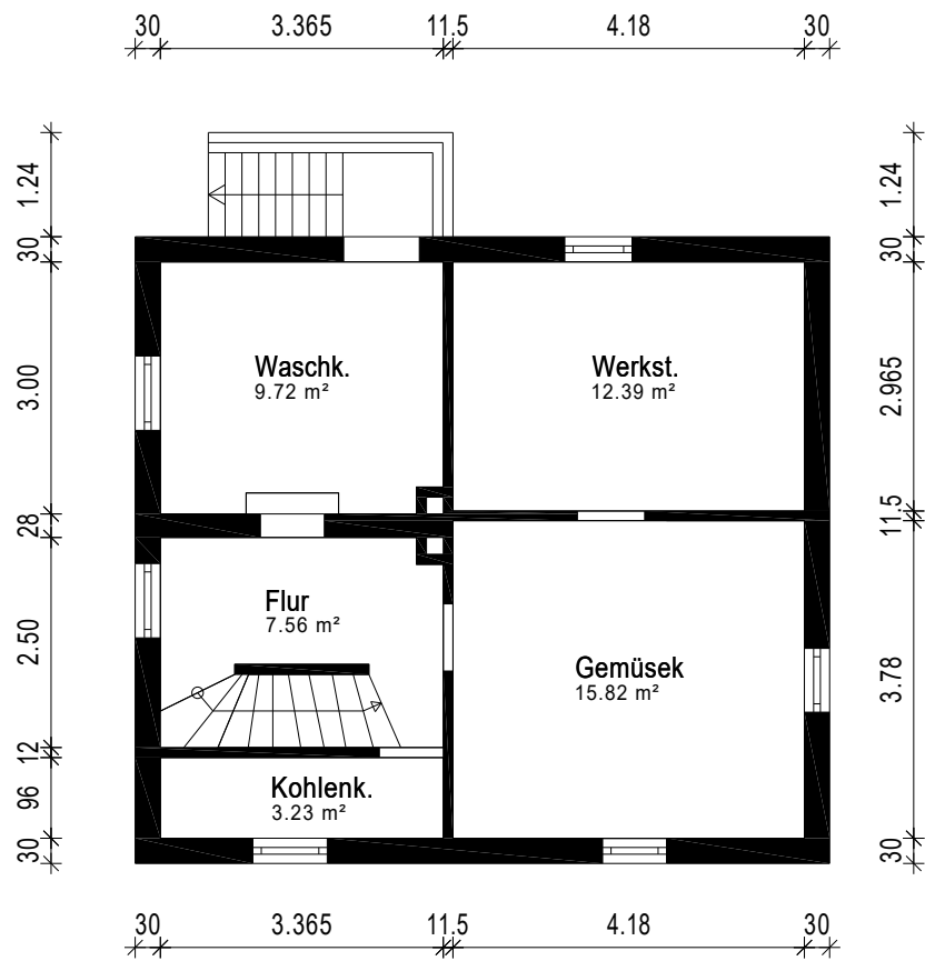
Kellergeschoss
