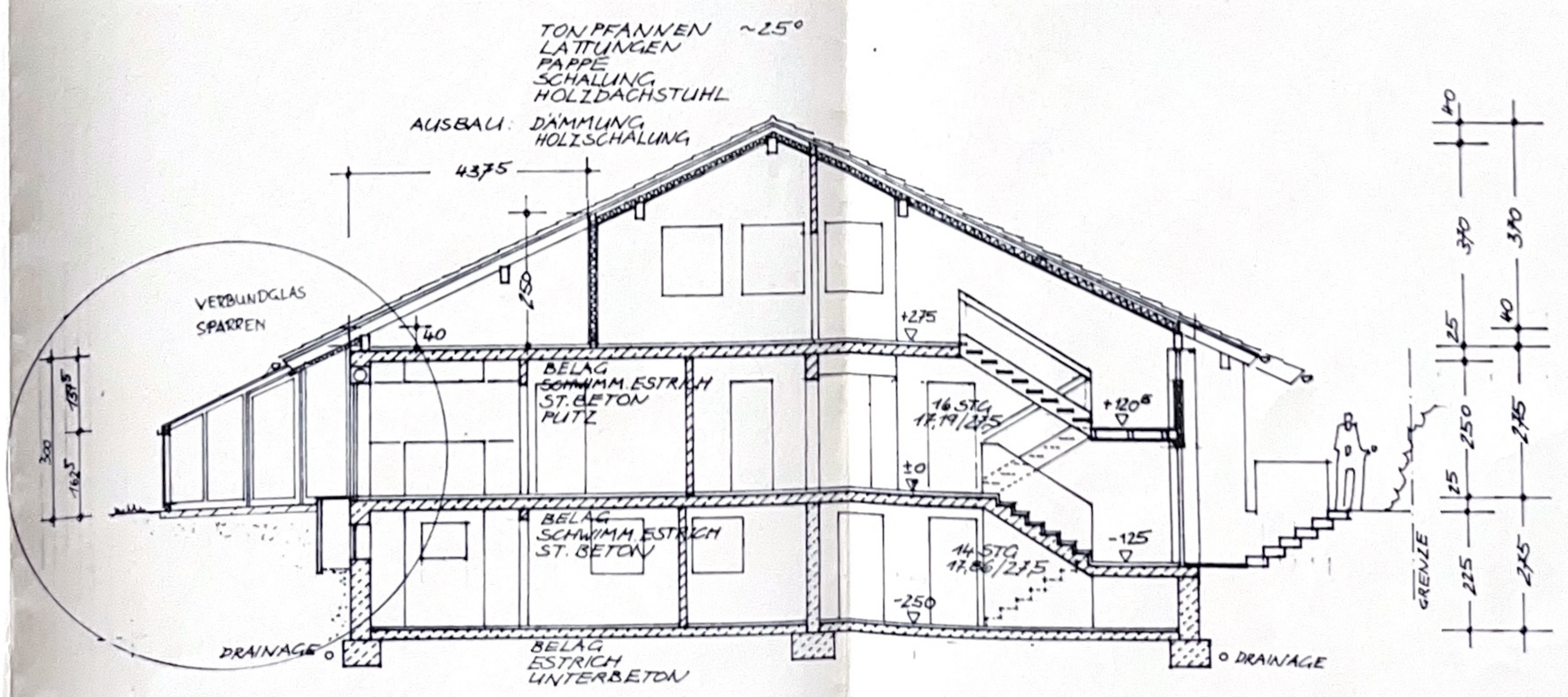
SCHNITT A
