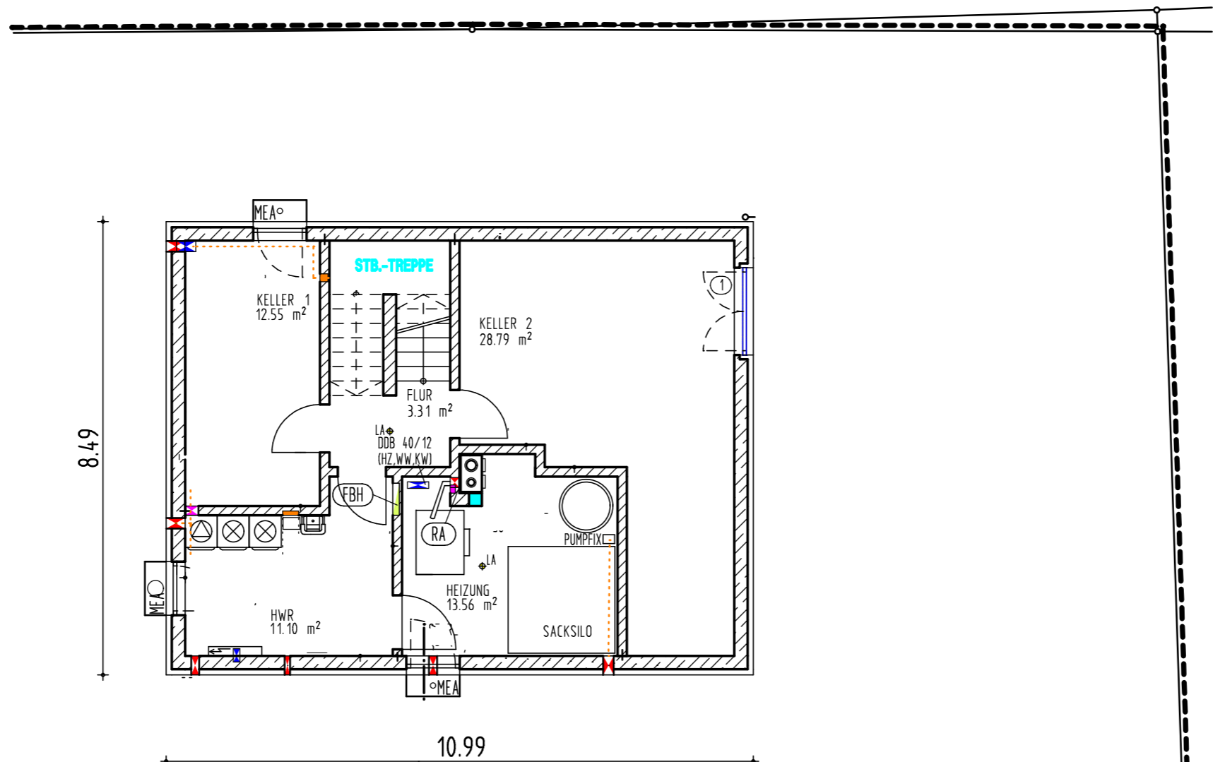
KELLERGESCHOSS
