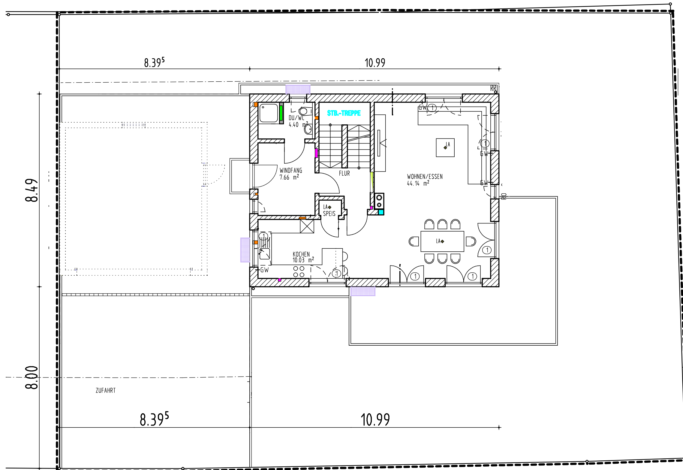
GRUNDRISS ERDGESCHOSS
