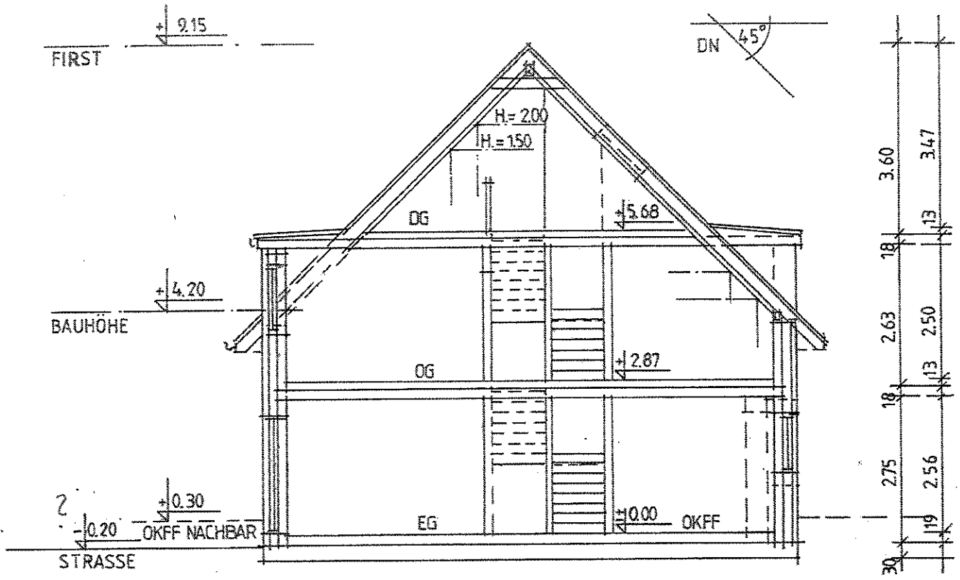
SCHNITT A-A
